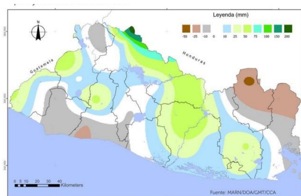
Figura 6. Perspectiva de la anomalía del acumulado de lluvia para junio 2025. Fuente: MARN-DOA-GMT.
