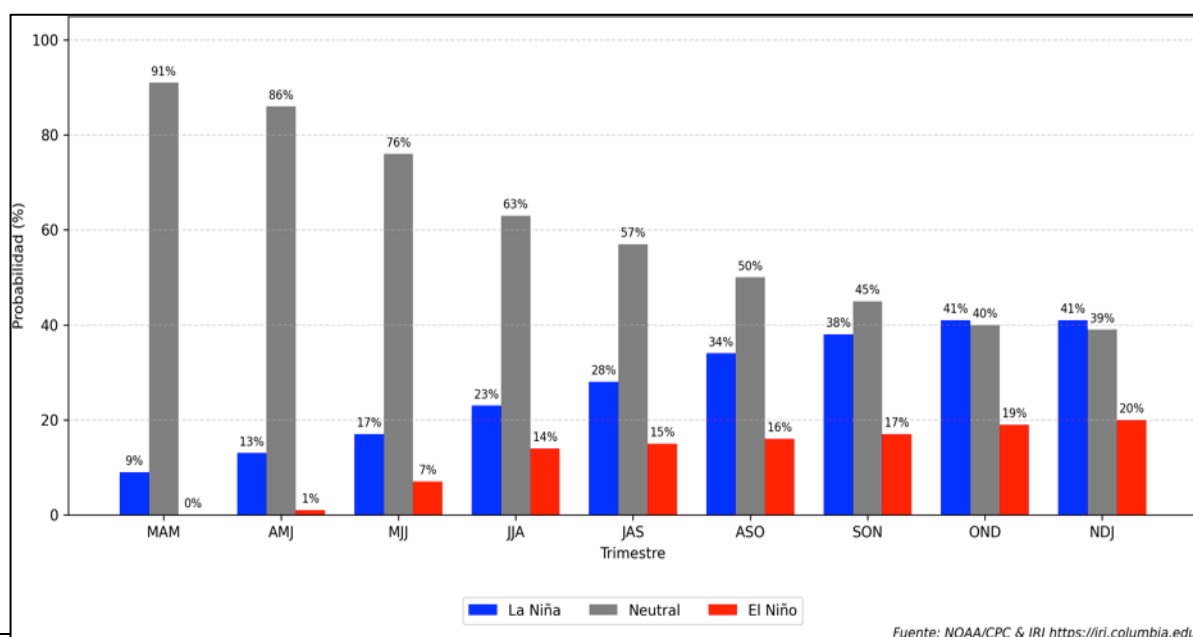
Figura 2. Pronostico probabilístico para el ENOS 2025. Fuente: NOAA CPC.
