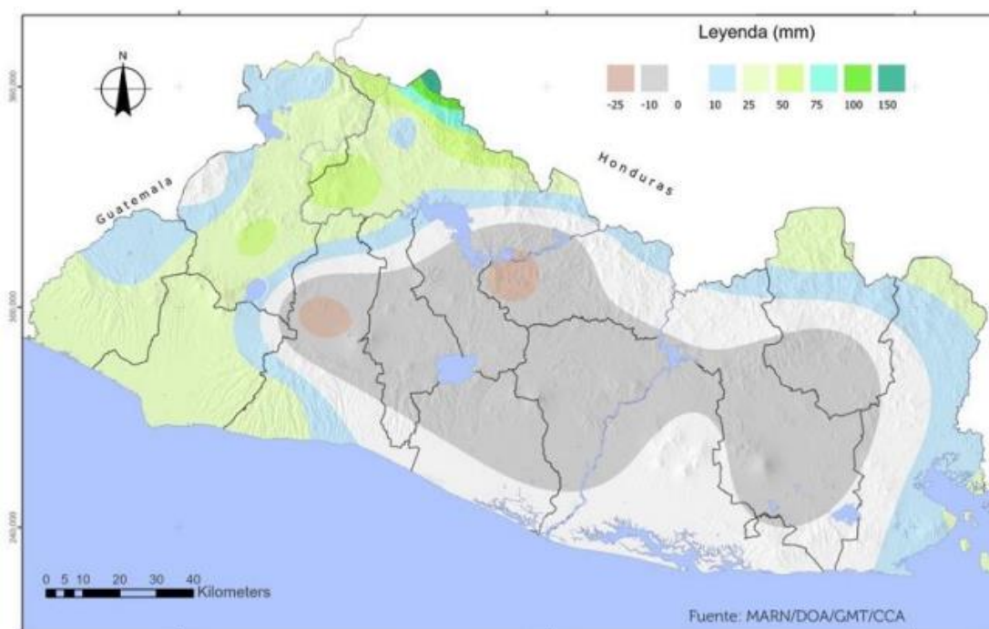
Figura 5. Perspectiva de la anomalía de lluvia acumulada para mayo 2025. Fuente: MARN-DOA-GMT
