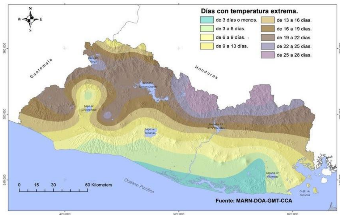
Figura 1. Número de días en que el umbral de la ola de calor fue superado entre el mes de marzo de 2025. Fuente: MARN- DOA-GMT.
