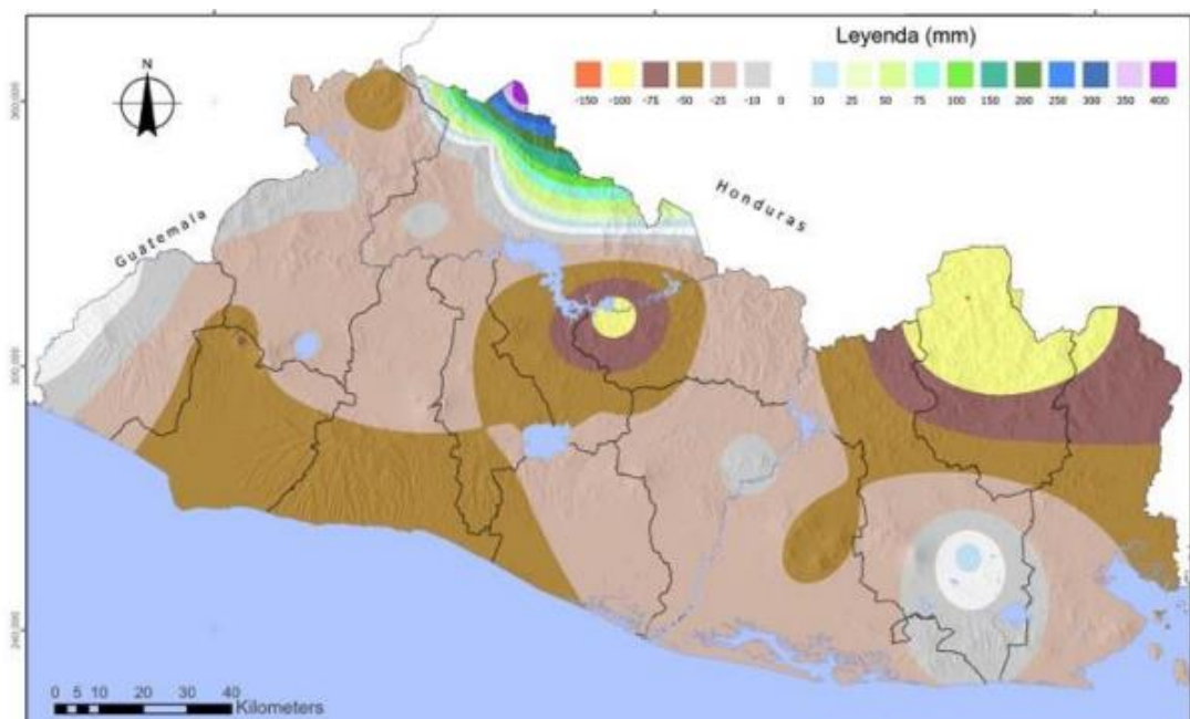
Figura 4. Perspectiva de anomalías de lluvia. Meses mayo a julio 2025. Fuente: MARN-DOA-GMT
