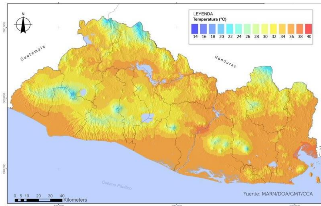
Figura 3. Perspectiva de temperatura máxima para trimestre mayo julio 2025. Fuente MARN/ DOA/GMT/CCA
